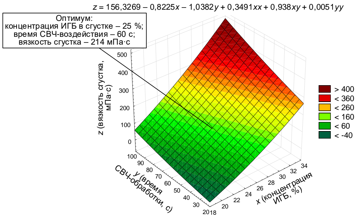
Рисунок 27 – Поверхность отклика зависимости вязкости белково-растительной основы эмульсий от концентрации ППБС и времени СВЧ-воздействия (на примере ИГБ)
